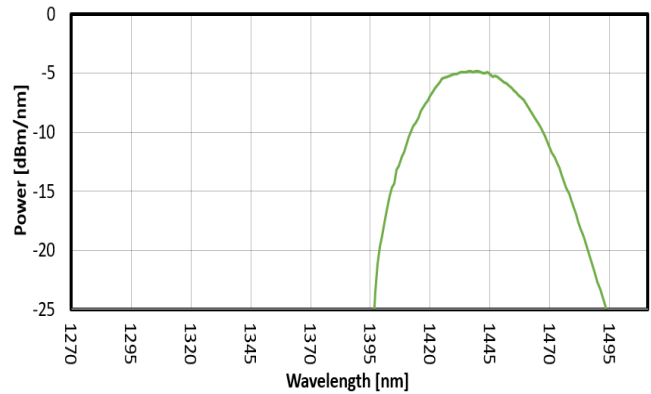
FIG. 2: SLED 1 SPECTRUM
