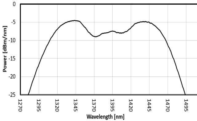
FIG. 1: OSE2 SPECTRUM
