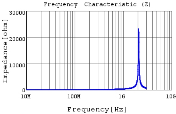
LQG15WZ39NG02 |Z|
