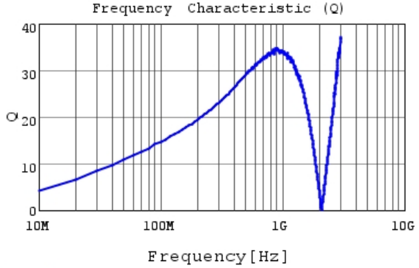
LQG15WZ39NG02 Q
