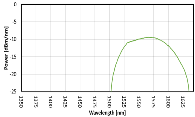
FIG. 2: SLED 1 SPECTRUM
