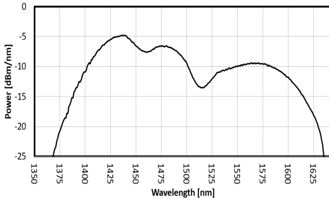
FIG. 1: OSE2 SPECTRUM
