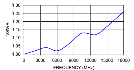
BW-S5W5+ VSWR
