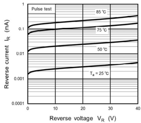
Fig. 9.2 I_R - V_R
