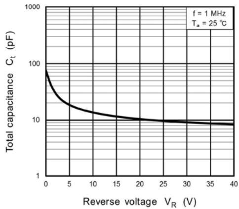
Fig. 9.3 C_t - V_R
