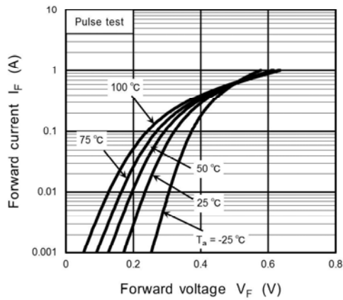
Fig. 9.1 I_F - V_F
