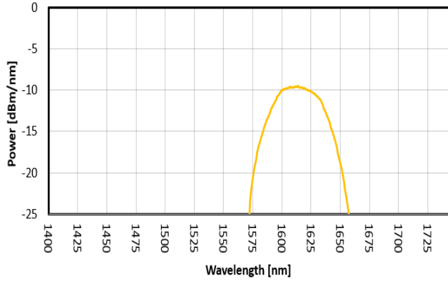
FIG. 3: SLED 2 SPECTRUM
