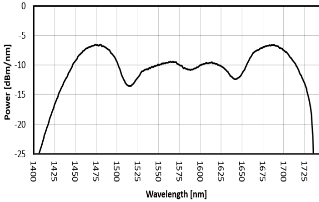
FIG. 1: ISB2 SPECTRUM
