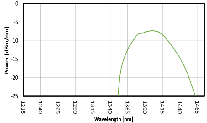
FIG. 4: SLED 3 SPECTRUM
