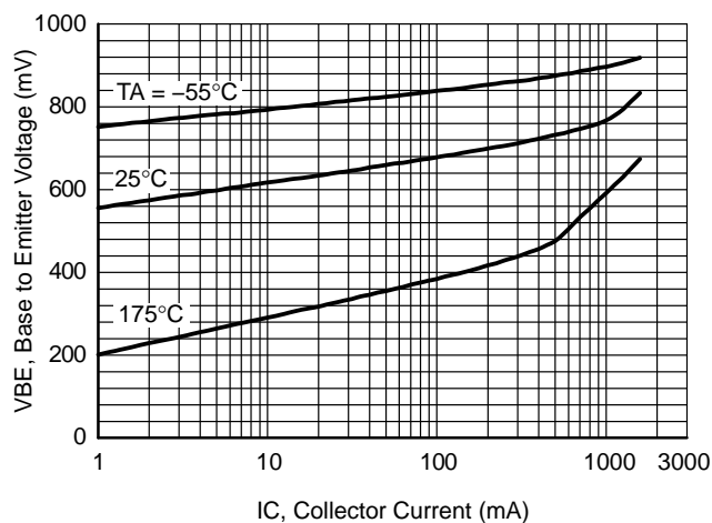
Figure 5. VBE – IC
