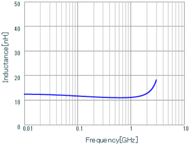
LQP02TN11NJ02 L.
