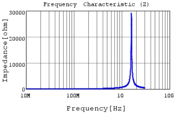
LQG15WZ68NG02 |Z|
