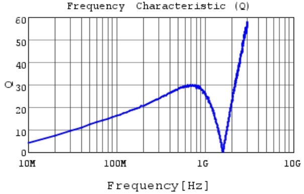
LQG15WZ68NG02 Q
