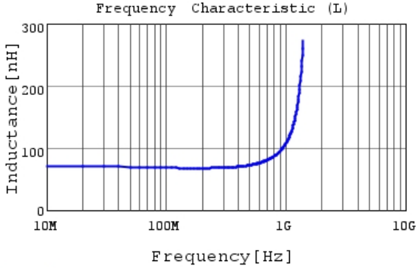
LQG15WZ68NG02 L
