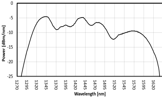
FIG. 1: ISB2 SPECTRUM
