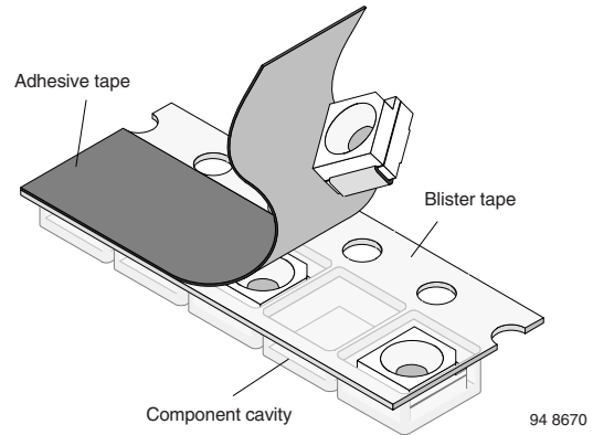
Fig. 12 - Blister Tape
