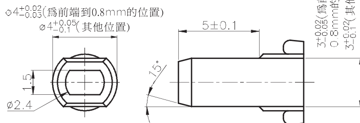
搖柄頭部尺寸(4:1)
