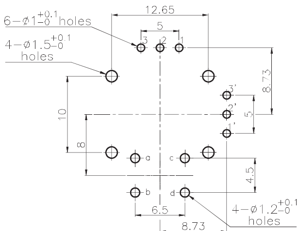
PCB板孔尺寸圖(2:1)
