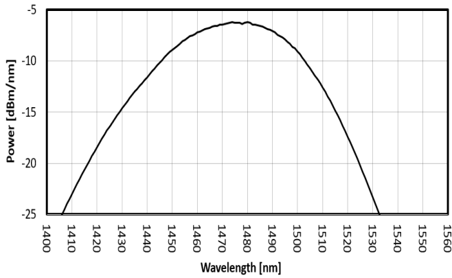
FIG. 1: ISB1 SPECTRUM
