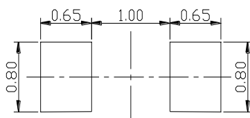
推荐焊盘尺寸
