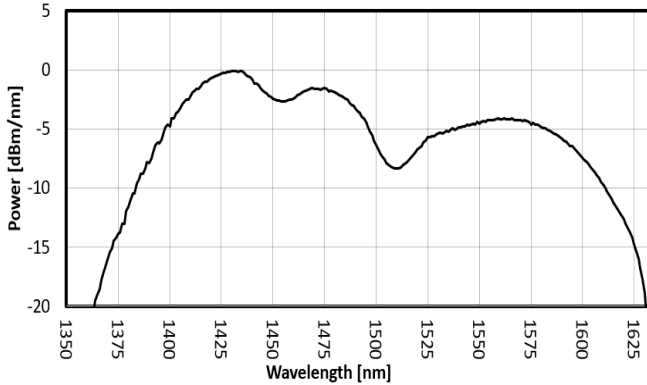
FIG. 1: ISB2 SPECTRUM
