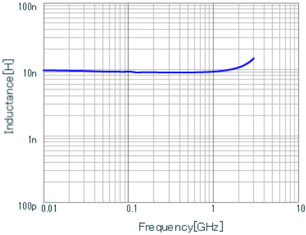
LQG15WZ9N1G02 L.
