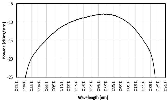
FIG. 1: ISB1 SPECTRUM
