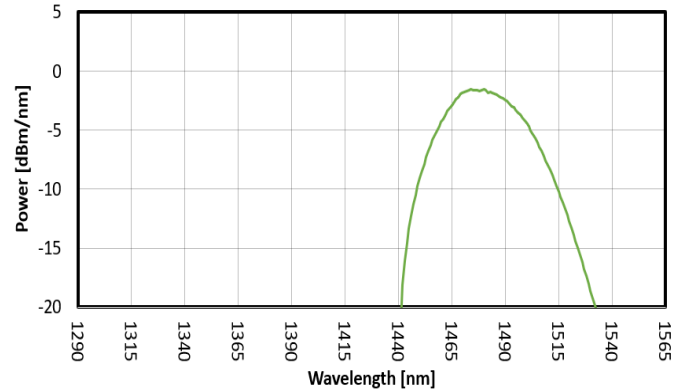
FIG. 4: SLED 3 SPECTRUM
