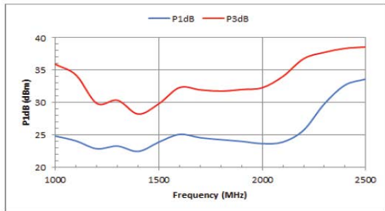
P1dB & P3dB
